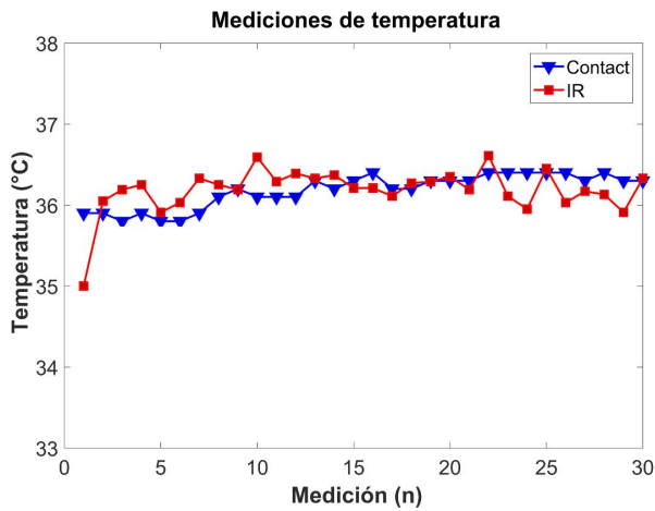
Fig. 8. Series de tiempo de las mediciones de temperatura del primer experimento obtenidas por ambos instrumentos de medición. Los datos del sensor IR de temperatura fueron compensación por el sesgo constante encontrado durante el análisis de Bland-Altman.
