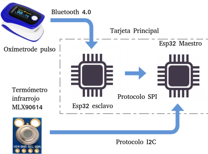
Fig. 2. Esquema de la electrónica (sistema embebido) incluido en el Kit Clínico. El Esp32 esclavo funciona como receptor Bluetooth. El Esp32 maestro realiza la conexión WiFi y la gestión del Esp32 esclavo.
