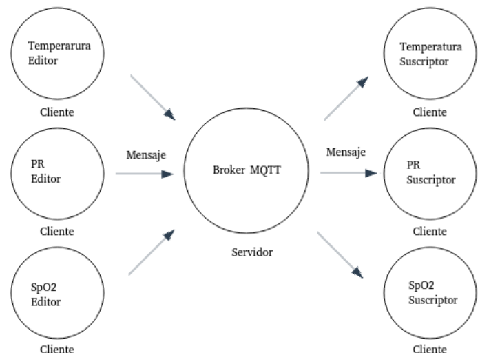
Fig. 3. Arquitectura IoT. Considera 3 tópicos: temperatura, frecuencia de pulso (Bpm) y nivel de oxigenación (SpO2).
