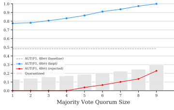
(a) AUT( F_1 , 48m)
