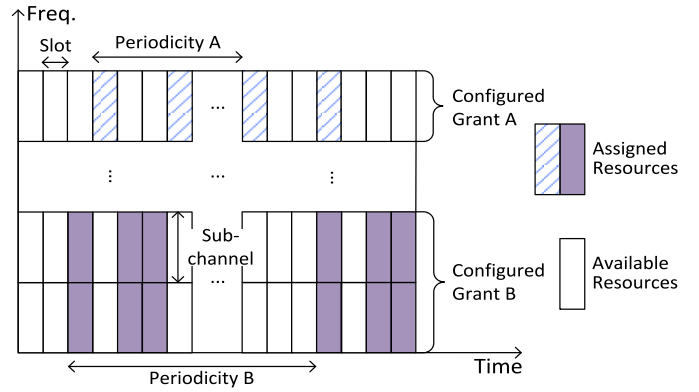
Fig. 16. Examples of CGs under NR V2X SL mode 1.
