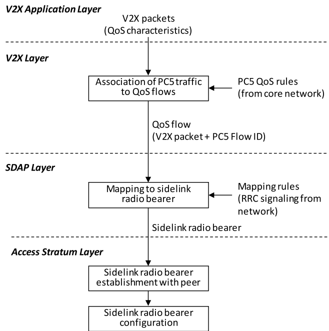
Fig. 21. Per-flow 5G QoS Model.
