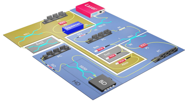
(d) QSDC relying on squeezed state [336]. © Paparella et al. arXiv, 2023.
