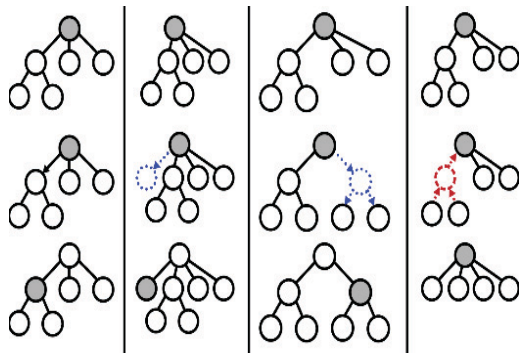
Fig. 3. COBWEB
