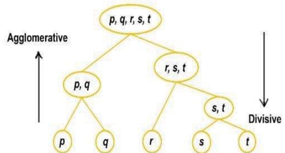
Fig. 6. Hierarchical Clustering
