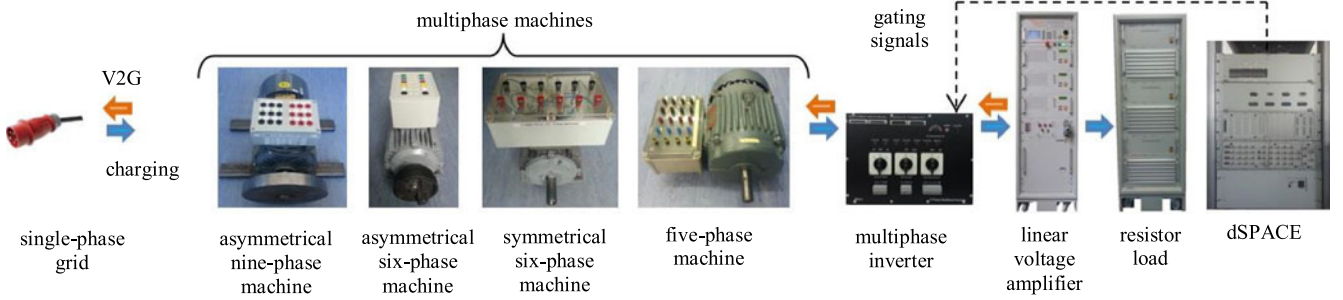
Fig. 7. Experimental rig.
