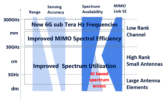
FIGURE 6. Spectrum options for 6G.
