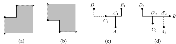
FIGURE 6. (a) BOTTOM_ORIENT. (b) TOP_ORIENT. (c) BOTTOM_ORIENT segment. (d) TOP_ORIENT segment.
