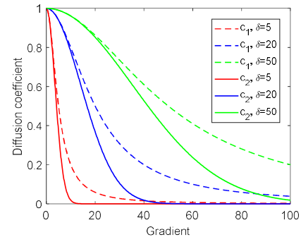
Fig.1. Diffusion function.
