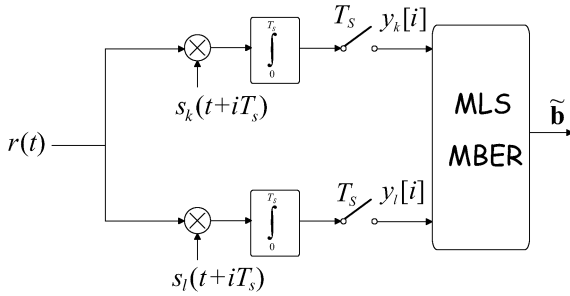
Fig. 19. Multiuser DS-SS detector.
