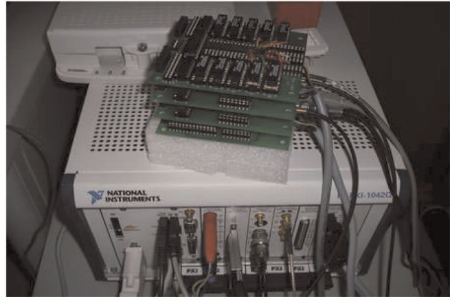
Fig. 7. VISIR-DEUSTO.
